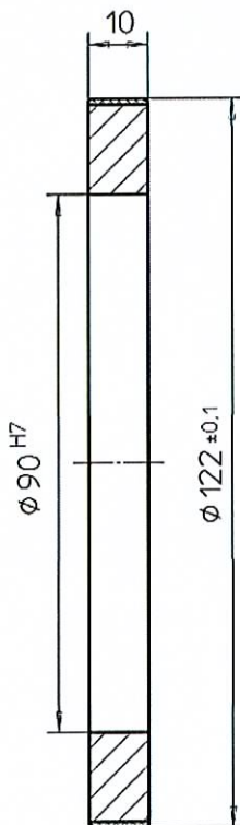
50802-KR117 Innendurchmesser variabel
