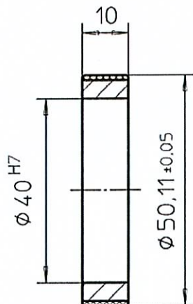
50770-KR108 Innendurchmesser variabel
