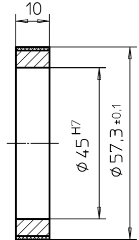
Innendurchmesser variabel
