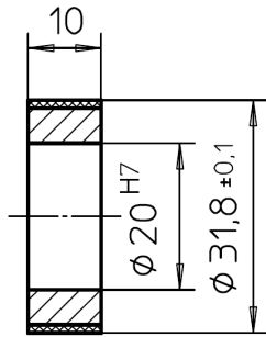
Innendurchmesser variabel
