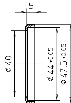
Innendurchmesser fix
